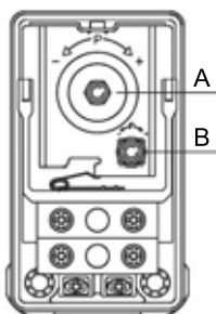
Rys. 1 Łącznik ciśnienia
